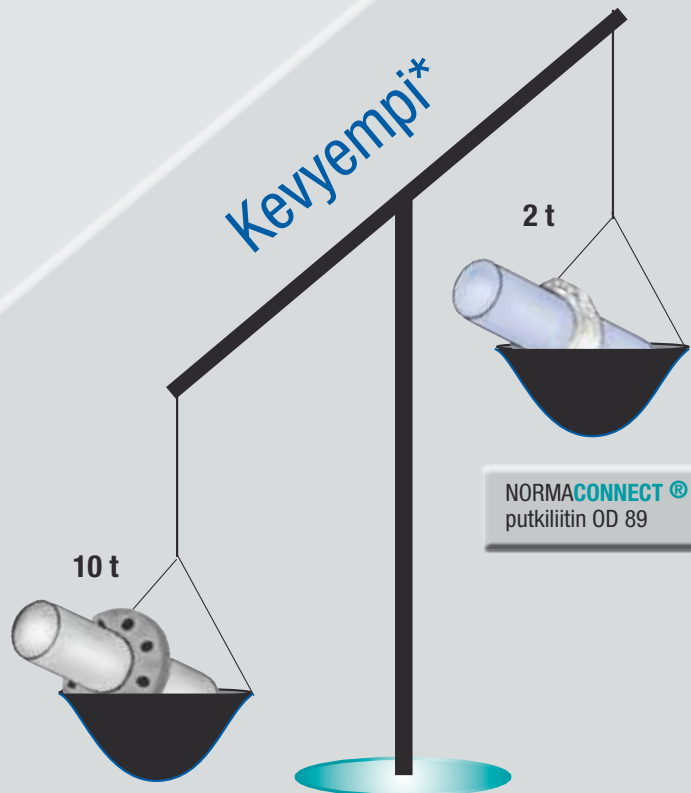
Laippaliitos OD 89
